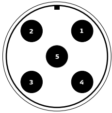
A) 5-napainen M12-urosliitin
