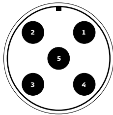
B) 5-napainen M12-urosliitin
