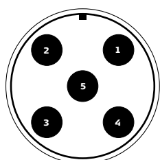
A) M12 hane, 5 stift
