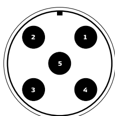
B) M12 hane, 5 stift
