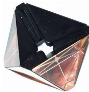
Abbildung 5 – Sechs Tripelprismen-Glaskörper
