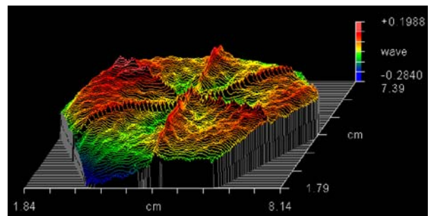
Abbildung 9 - Interferometermessung zur Bestimmung der Phasenheterogenität der reflektierten Strahlen (wie gut ist das jeweilige Prisma poliert)
