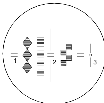
Retículo colimador modelo 727043
